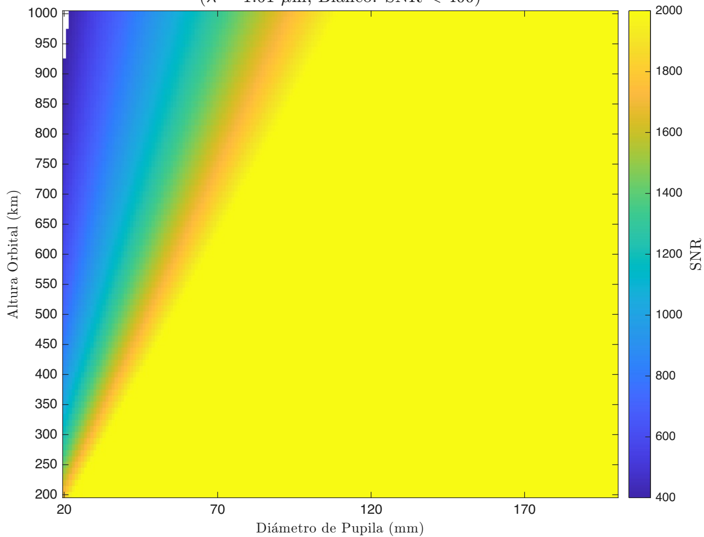
SNR - TMA - Detector 1 ( \lambda = 1.61 \mu\text{m} , Blanco: SNR < 400)
